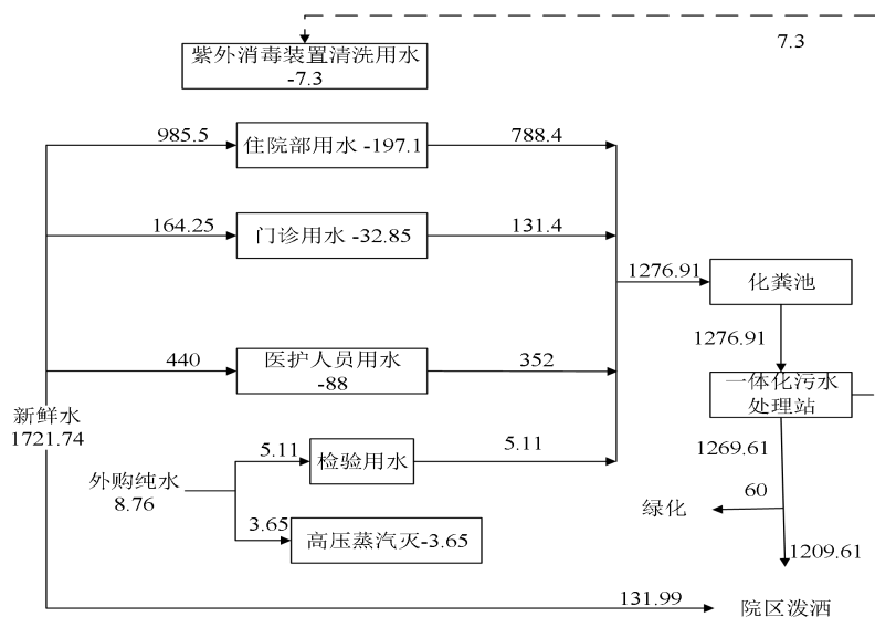
图3.5-1 项目给排水平衡图 单位：m³/a
