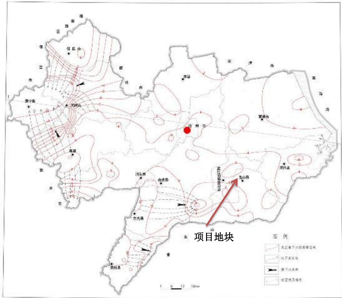
图 3-9 区域浅层地下水流向示意图
