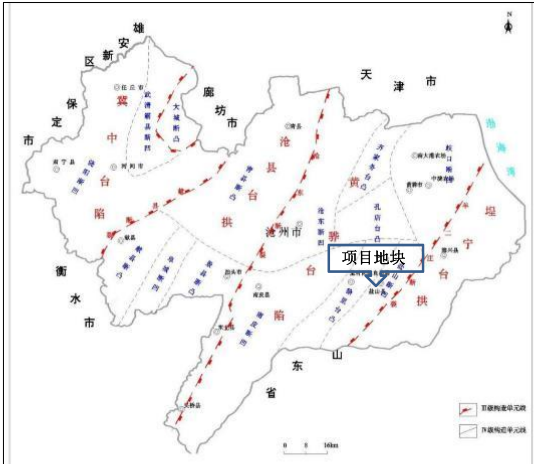
图 3-7 区域地质构造
